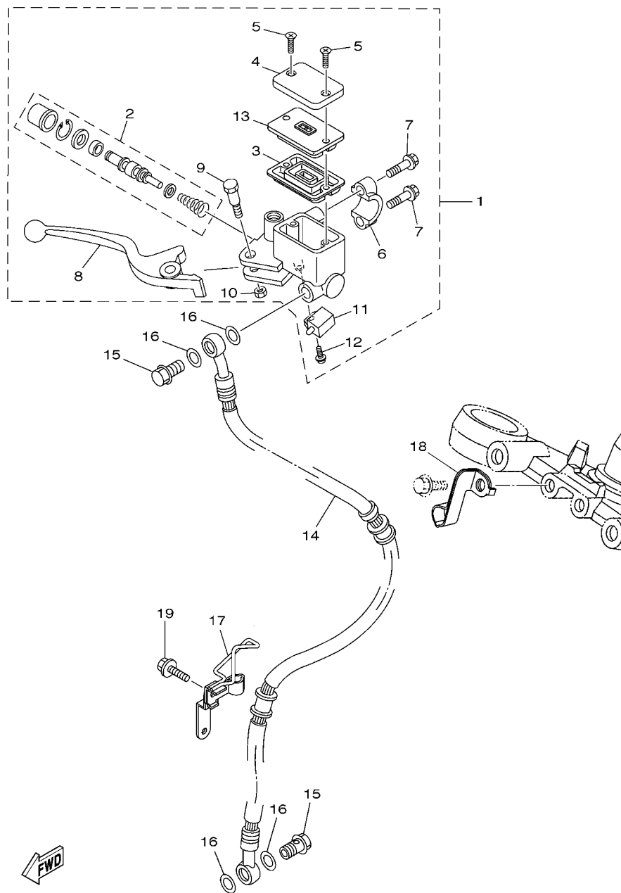
FIG. 31 CILINDRO MAESTRO DELANTERO
